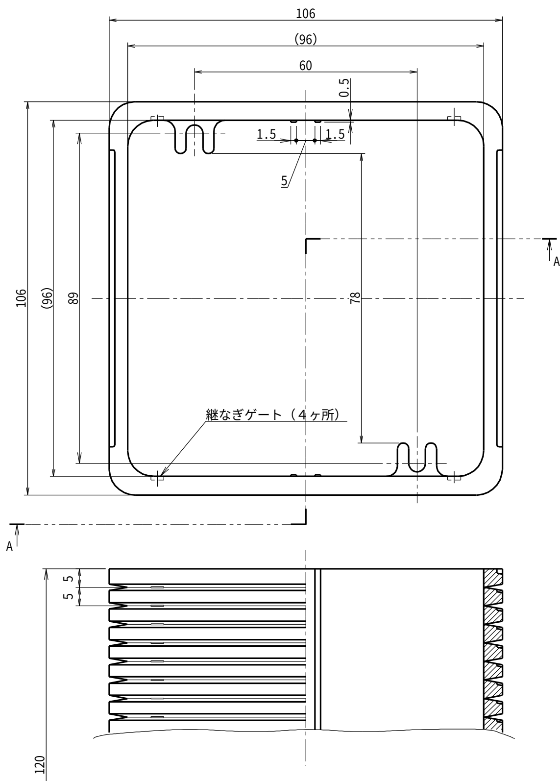
A-A断面図
